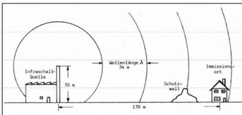
Ausbreitung einer Infraschallwelle bei 10 Hz – Dimensionsvergleich -
